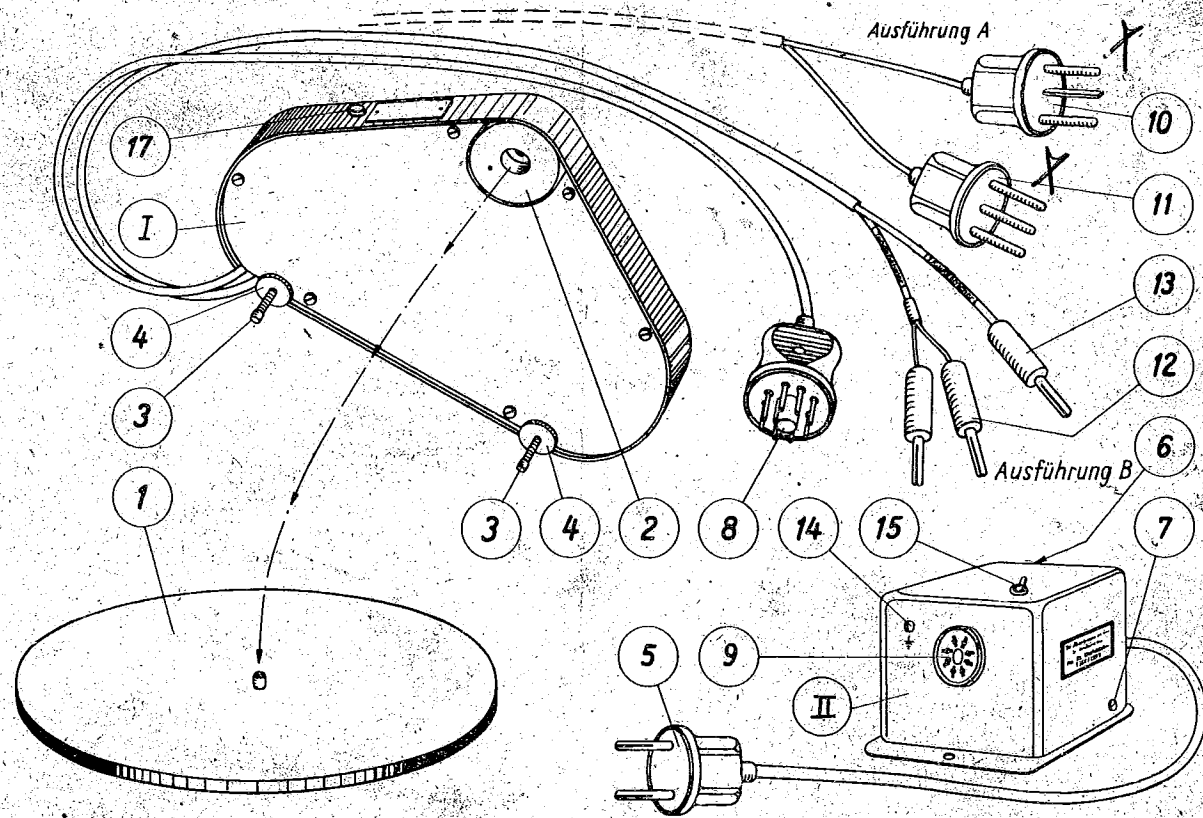
Anweisung für das Aufstellen und Anschließen des Gerätes.
